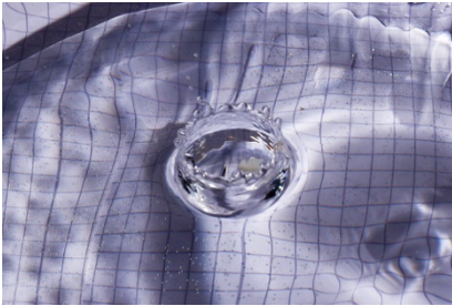
Gekrümmte Raum-Zeit?
